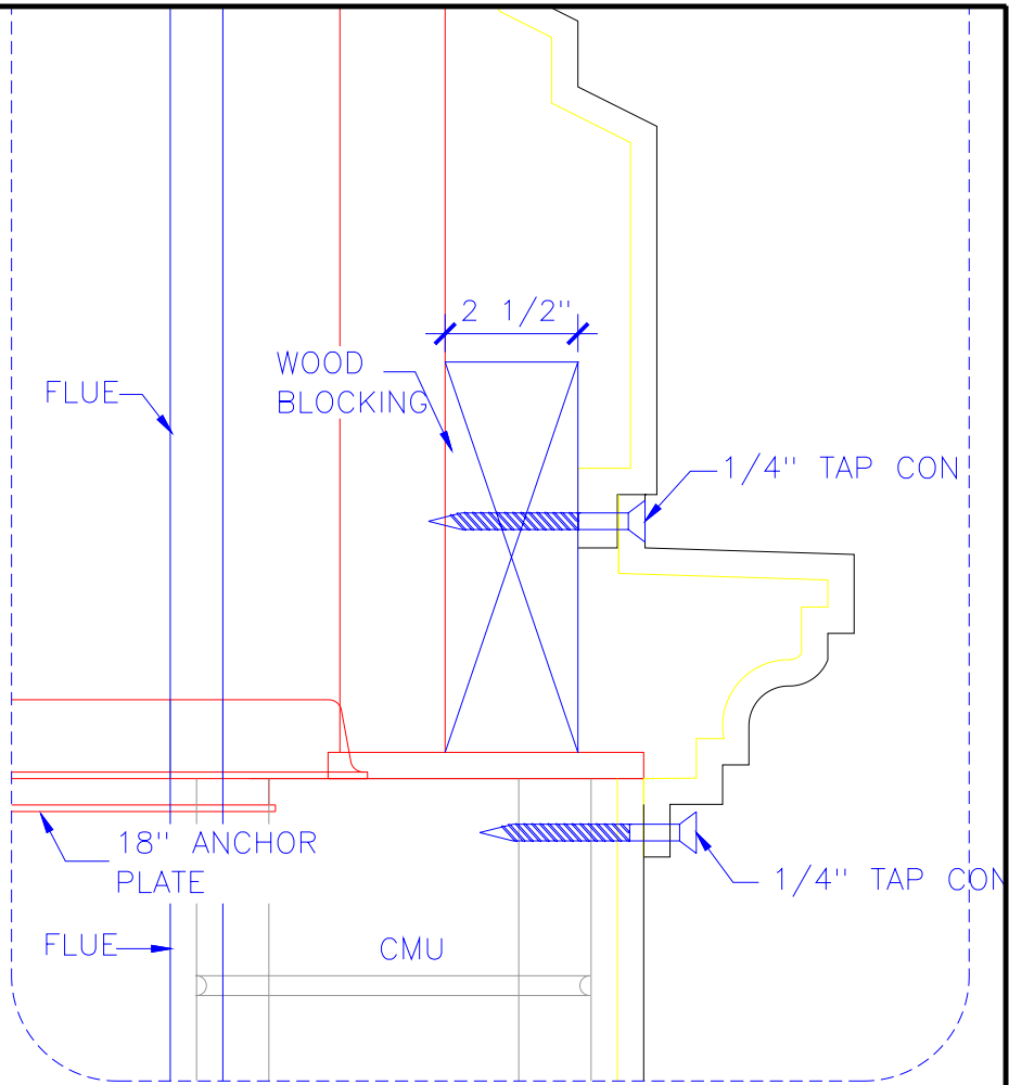
DETAIL B SCALE: 3" = 1'
