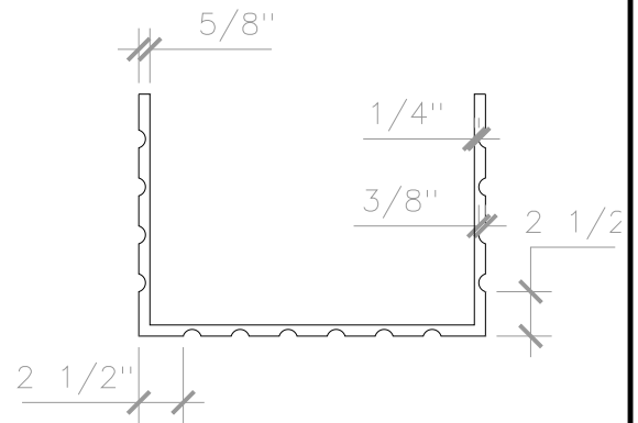
SECTION A (2X)
