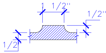
SECTION A SCALE: 3" = 1'
