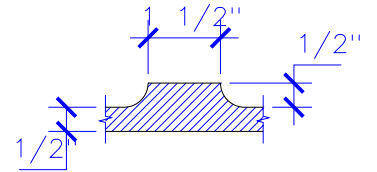
SECTION A SCALE: 3" = 1'
