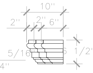
SECTION A SCALE: 1 1/2" = 1'
