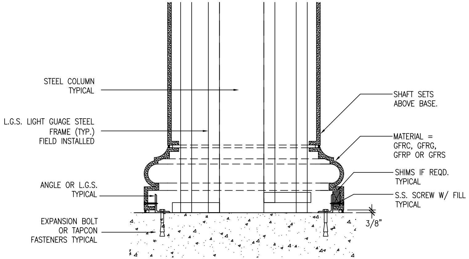
SHAFT THRU BASE SCALE: 1 1/2" = 1'-0"
