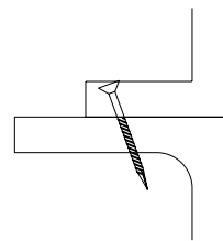
DETAIL D SCALE: 4" = 1'
