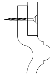
DETAIL C SCALE: 4" = 1'
