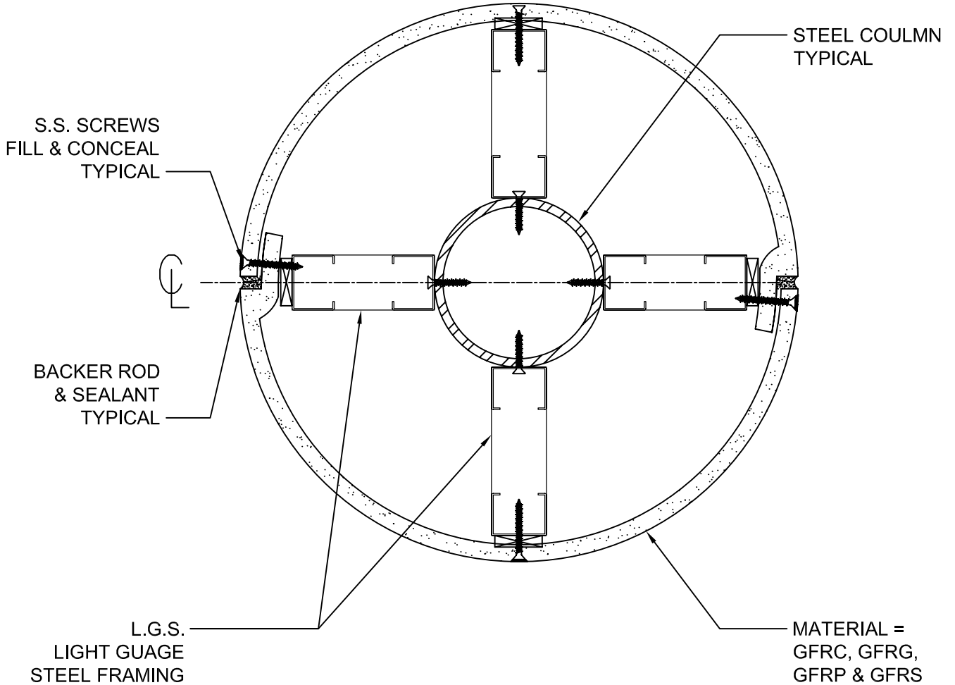
TYP COLUMN SECTION SCALE: 3" = 1'-0"
