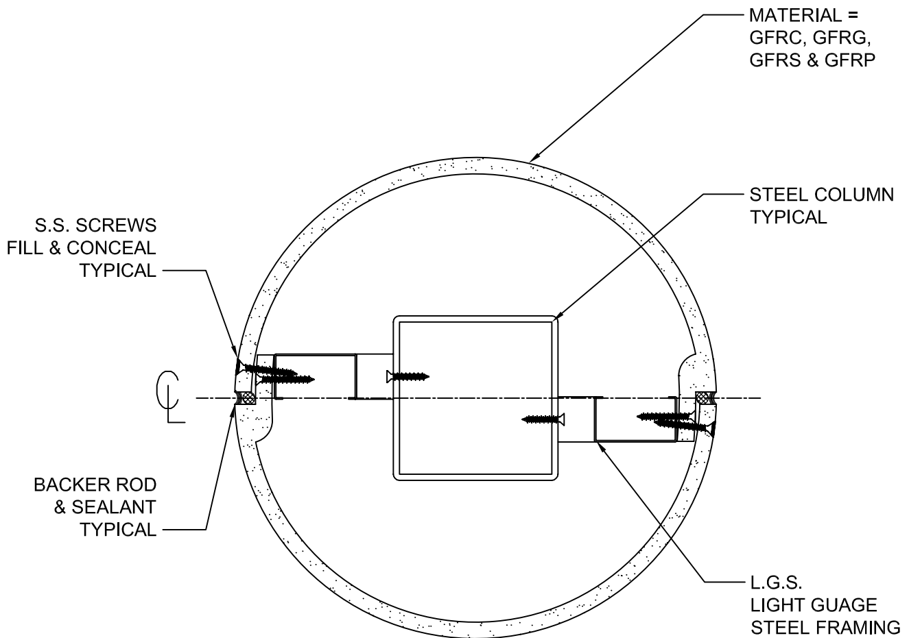
SECTION A SCALE: 3" = 1'-0"
