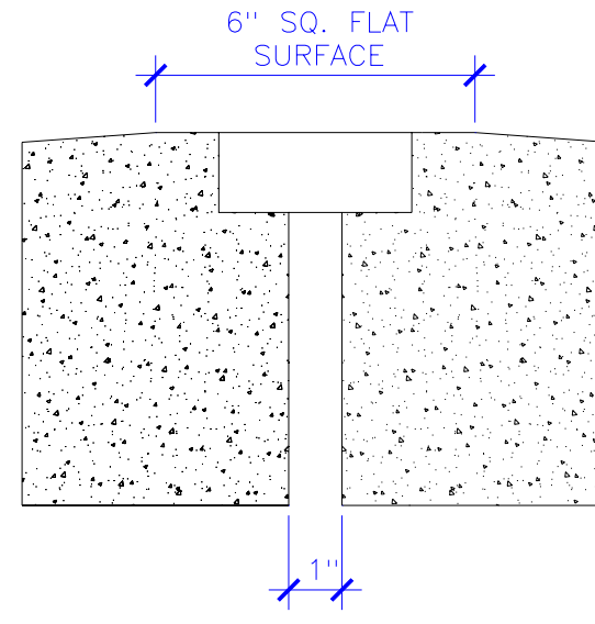
SECTION A SCALE: 3" = 1"
