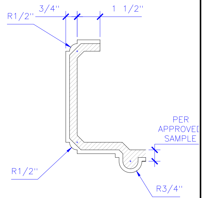
SECTION A SCALE: 3" = 1'
