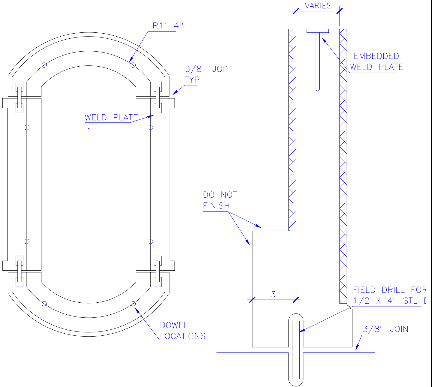
WALL DETAILS SCALE: 3" = 1'
