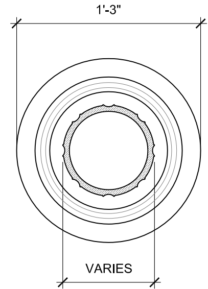
SECTION B SCALE: 1 1/2" = 1'-0"
