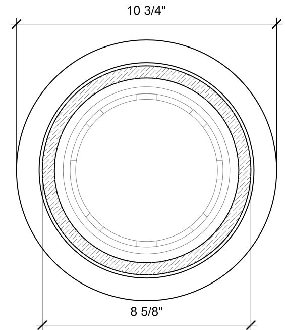
SECTION B SCALE: 3" = 1'-0"
