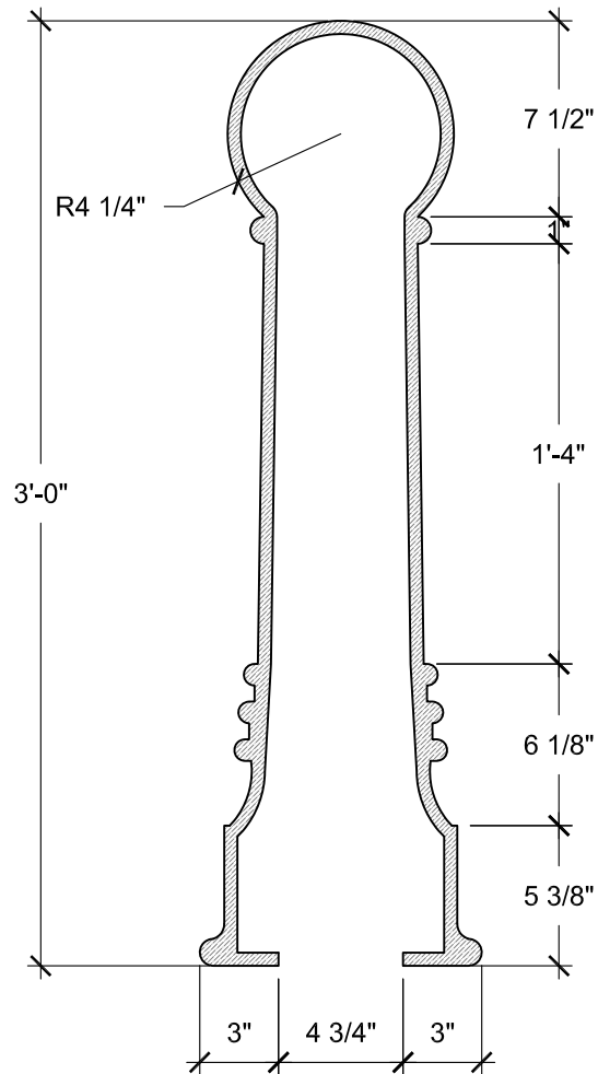
SECTION A SCALE: 1 1/2" = 1'-0"
