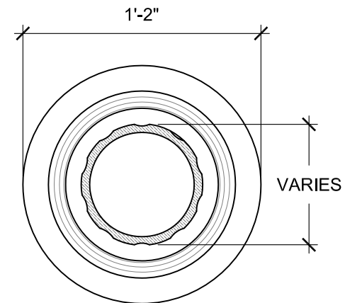
SECTION B SCALE: 1 1/2" = 1'-0"
