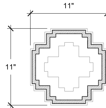
SECTION B SCALE: 1 1/2"= 1'-0"
