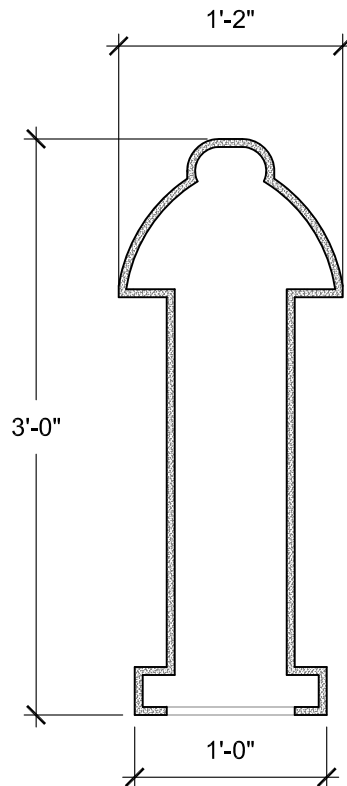
SECTION A SCALE: 1"= 1'-0"
