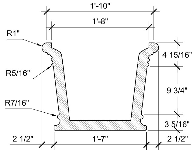
SECTION A SCALE: 1"= 1'-0"
