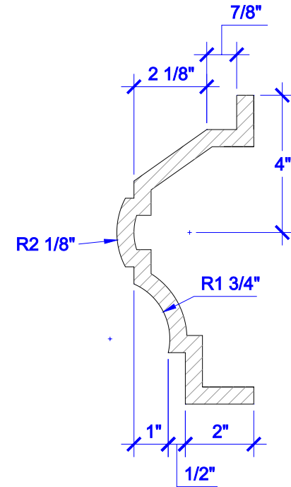
SECTION A SCALE: 3" = 1'
