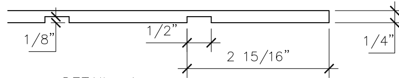
DETAIL A SCALE: 6" = 1'
