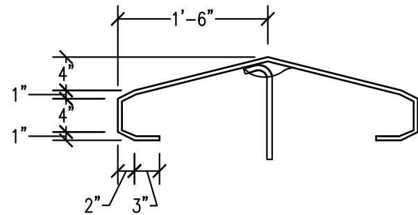
A F1 SECTION PROFILE
