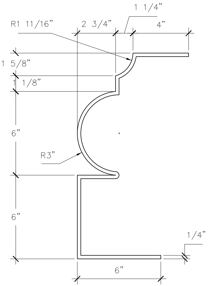
SECTION A SCALE: 3" = 1'
