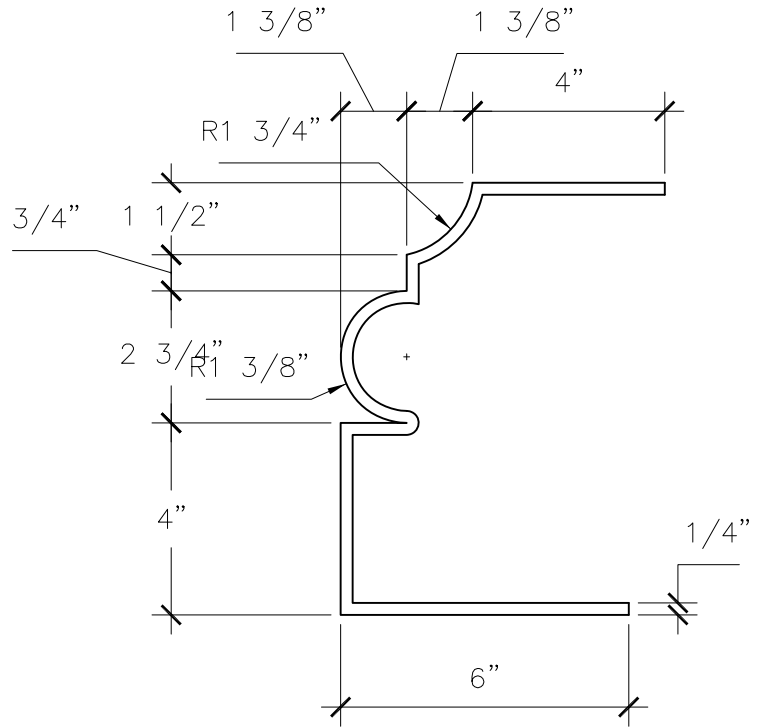
SECTION A SCALE: 3" = 1'
