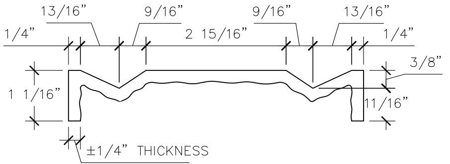
SECTION A SCALE: 6" = 1'
